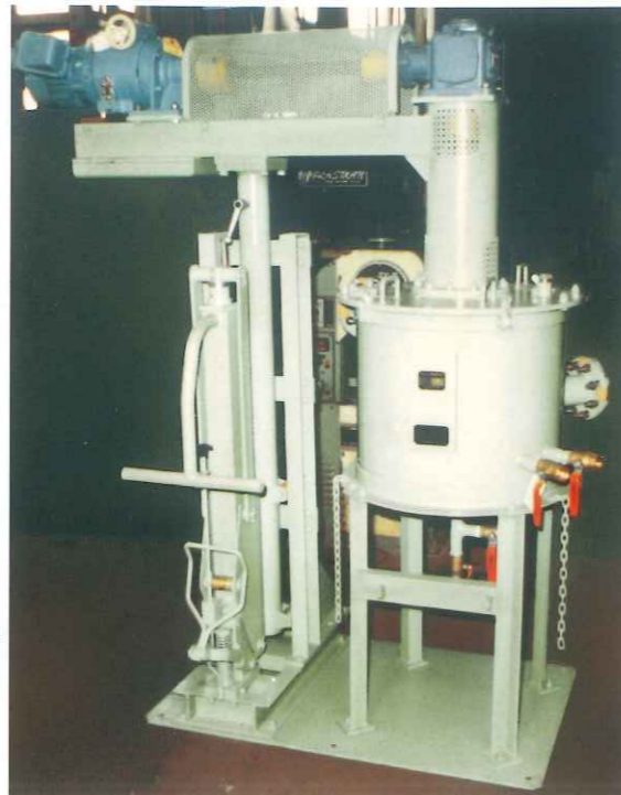
▼塗料混合槽
