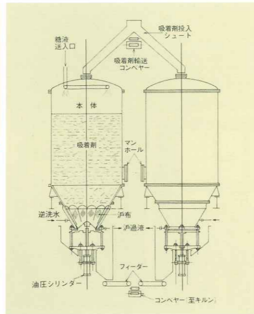
▲糖液濾過器
